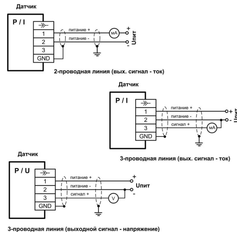
Рисунок 1 – Примеры схем подключения аналоговых выходов для разъема DIN 43650A
