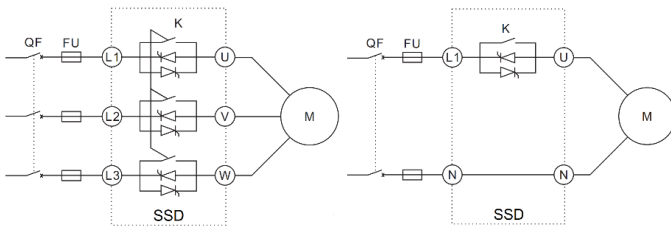
1. Для моделей с трехфазным питанием 2. Для моделей с однофазным питанием.
